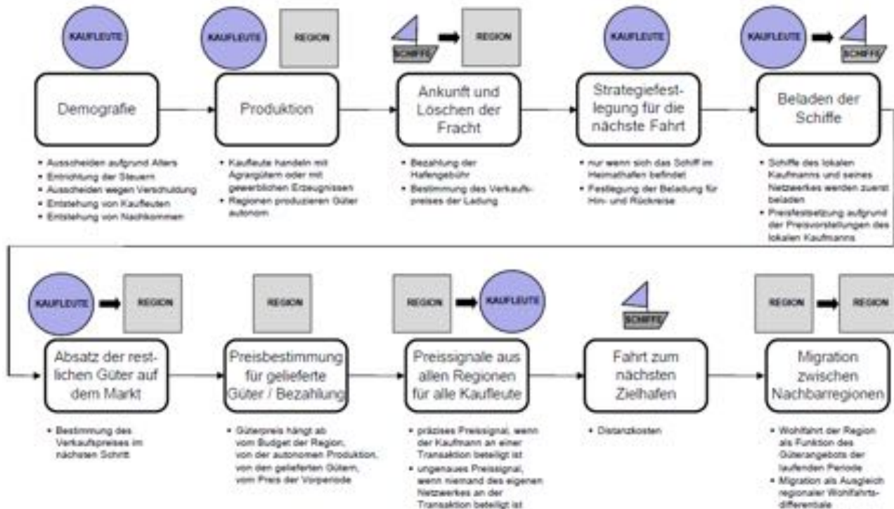
Abb. 1: Flussdiagramm einer Simulationsperiode des Multi-Agenten-Modells
